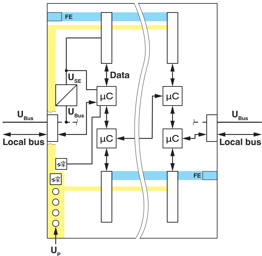
blokschema
