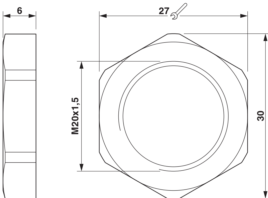
Maatschets
