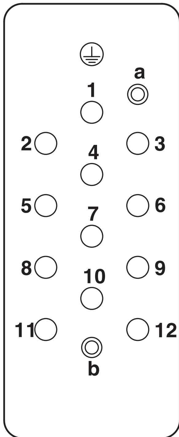
schematekening
