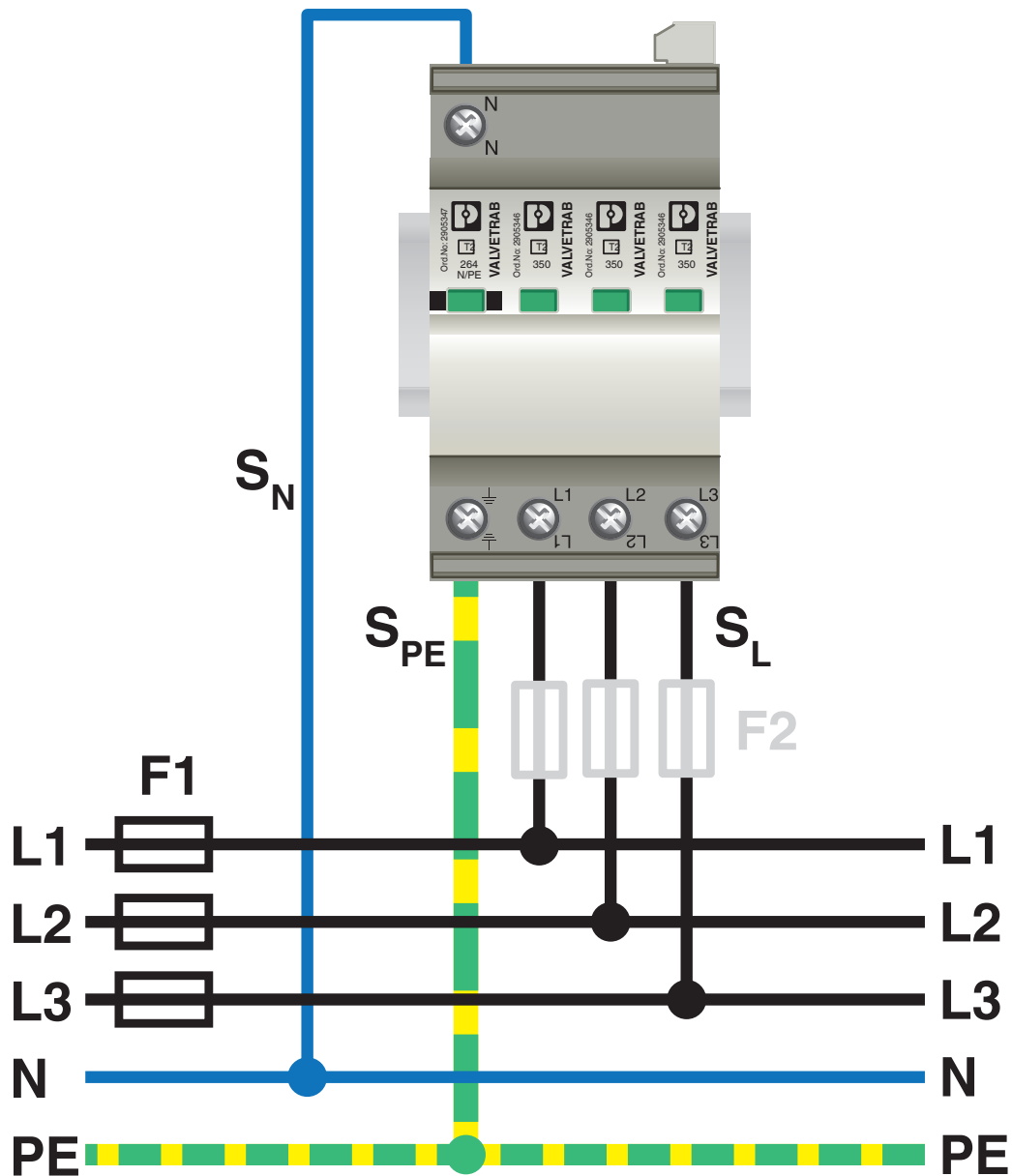
applicatietekening
