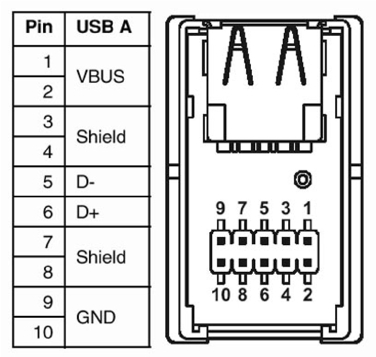
Contactbezetting
