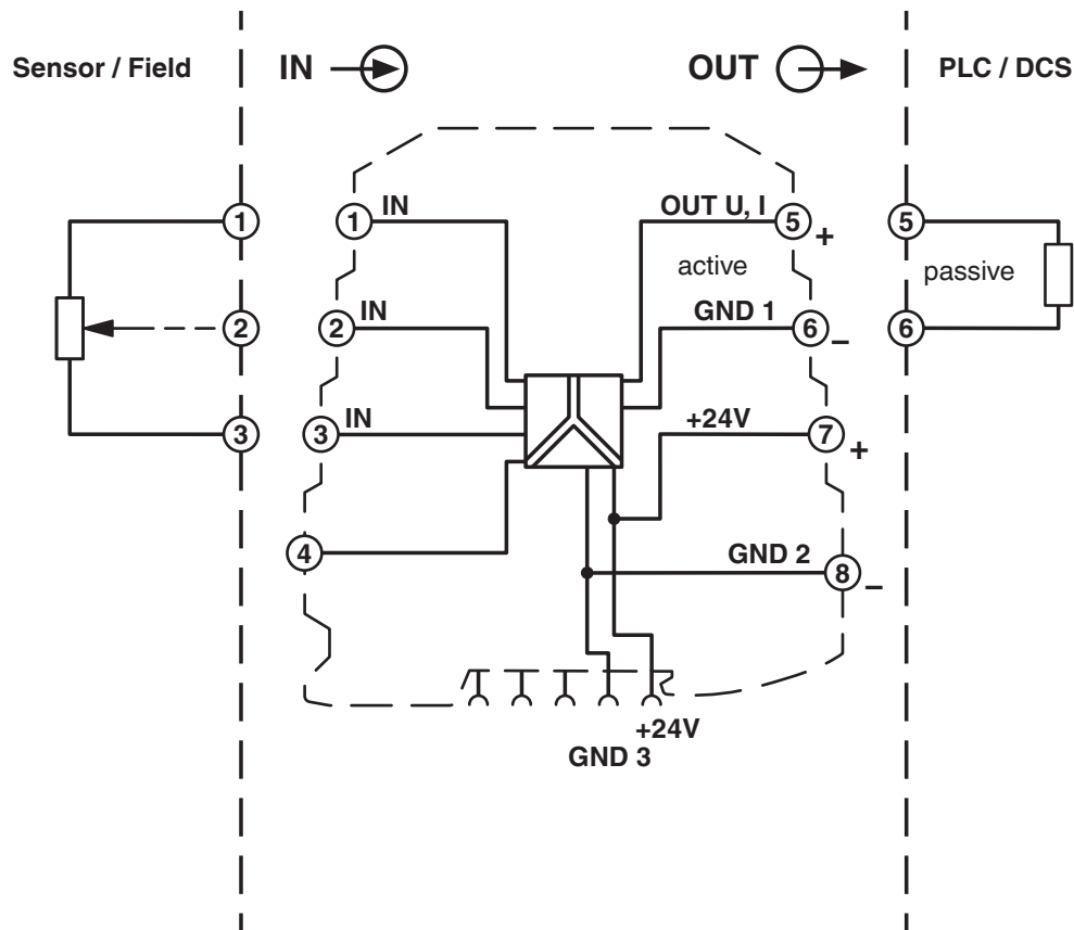
blokschema
