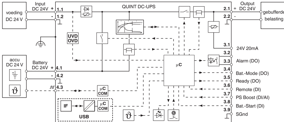
blokschema
