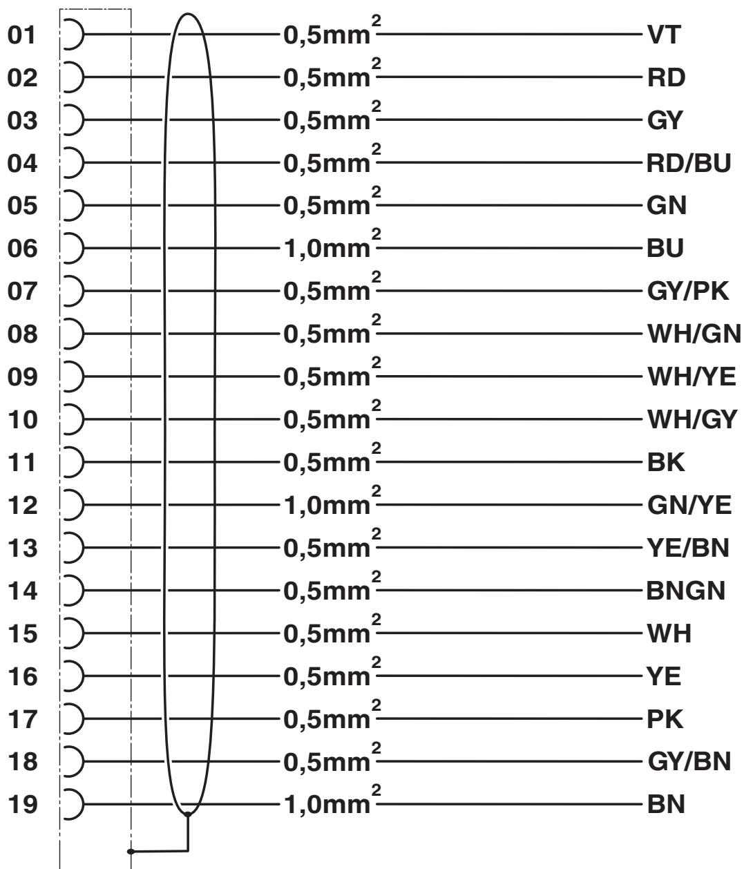
schakelschema
