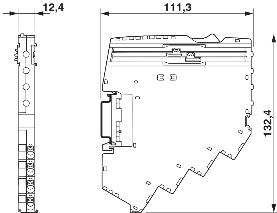
Producttekening
