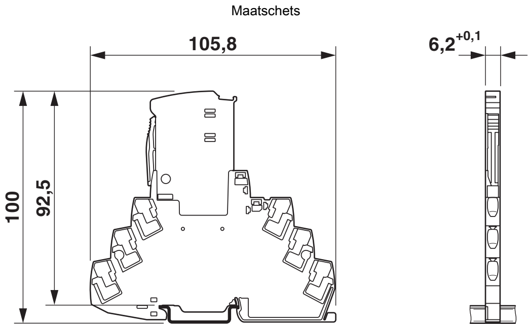
schematekening
