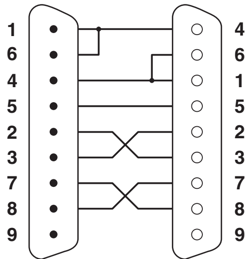
schakelschema
