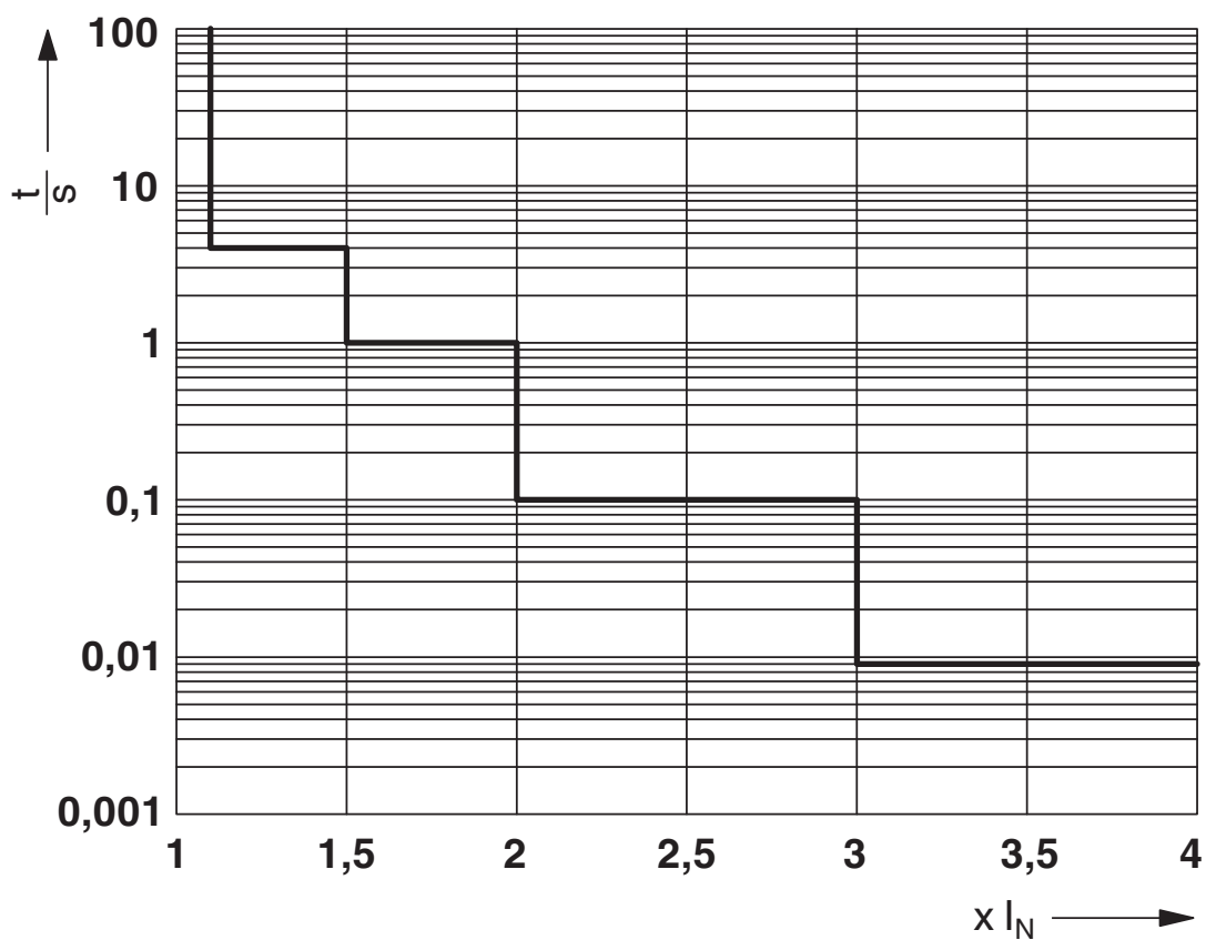
Uitschakelkarakteristiek
