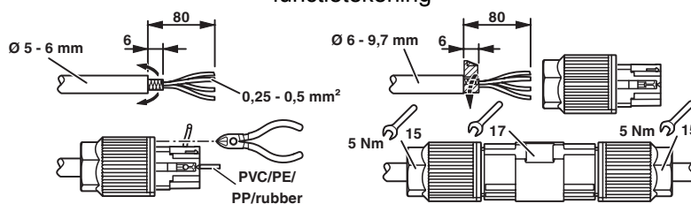
functietekening
