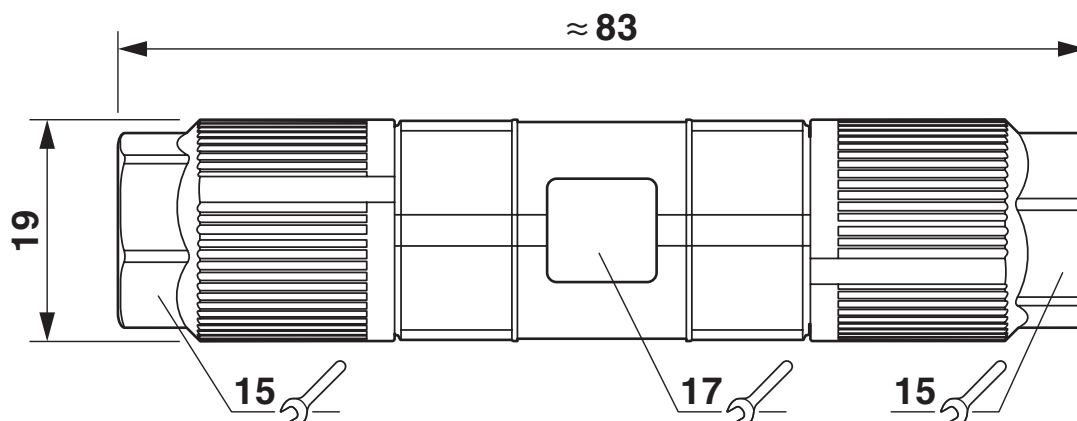
Maatschets
