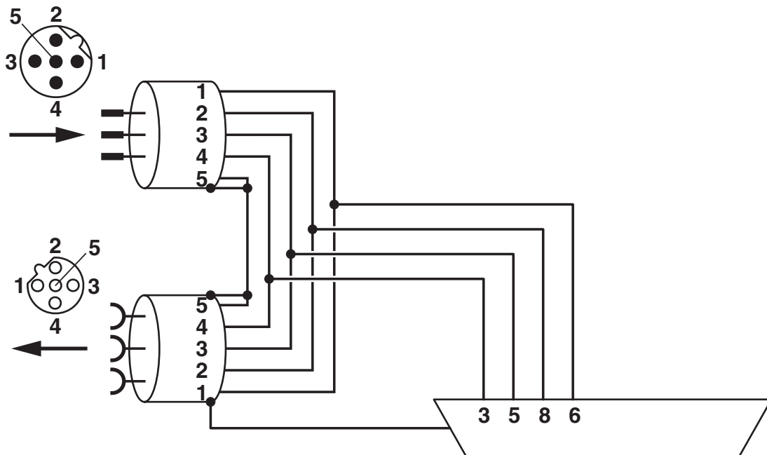
Functieschakelschema SUBCON-PLUS-PROFIB/...M12
