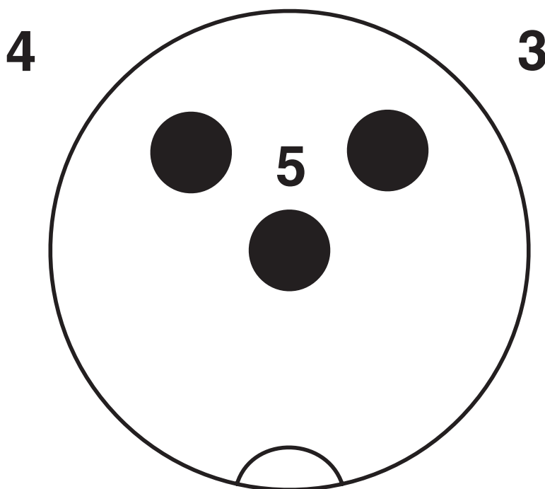
Poolschema stiftconnector M12, 3-polig, A-gepolariseerd, aanzicht stiftzijde
