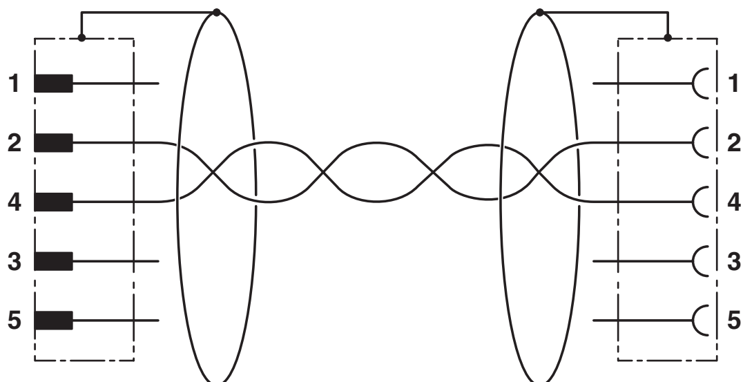
schakelschema
