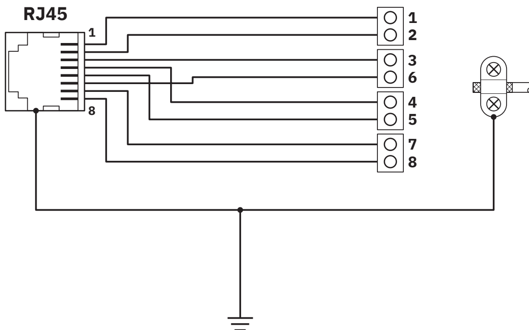
schakelschema
