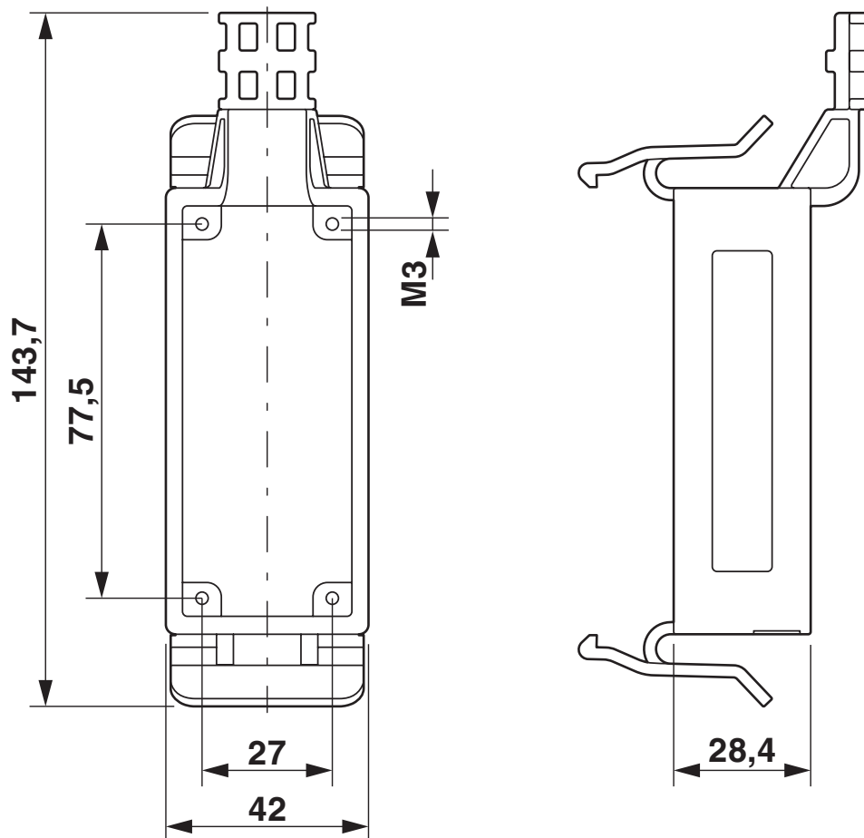
Maatschets
