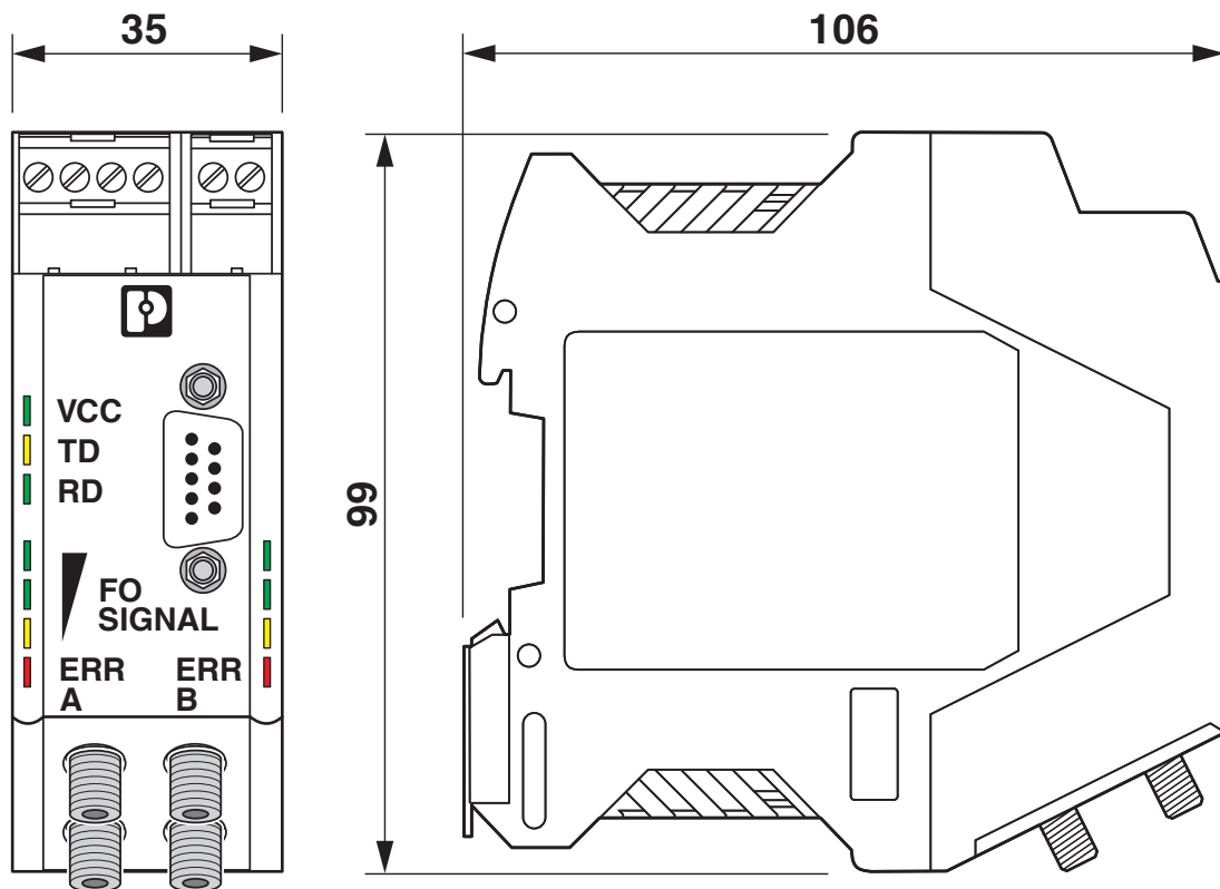
Maatschets
