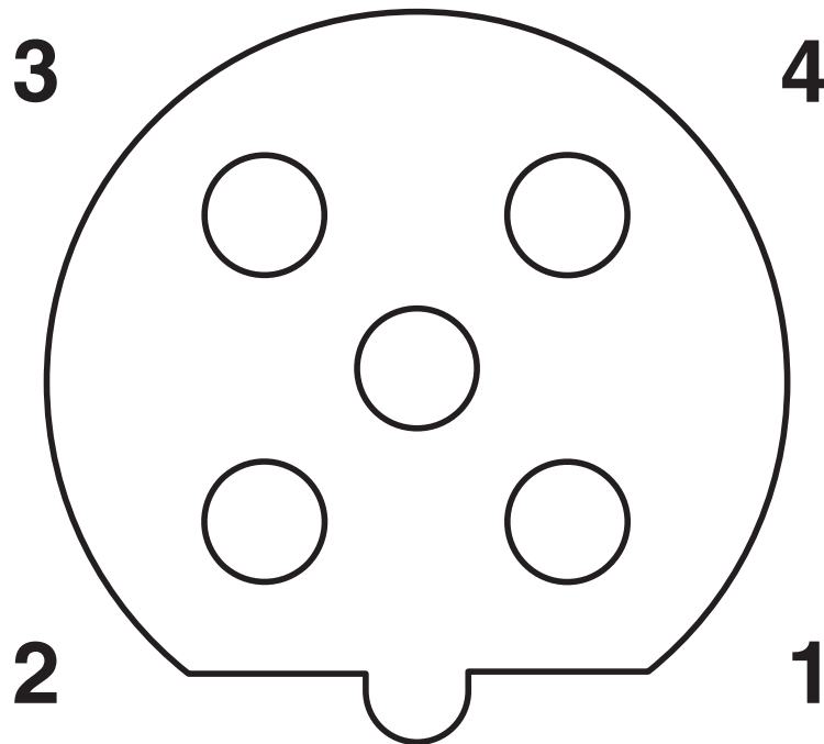
Poolschema bus M12, 5-polig, B-gepolariseerd, buszijde
