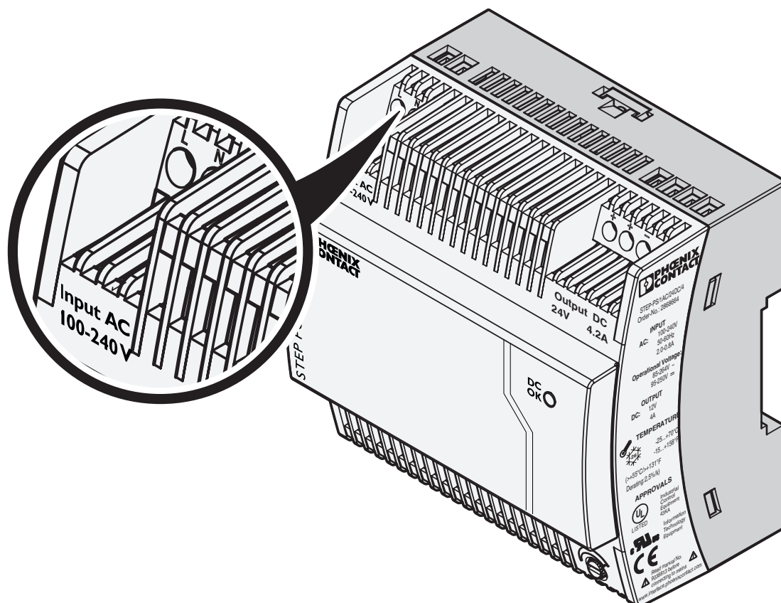
schematekening
