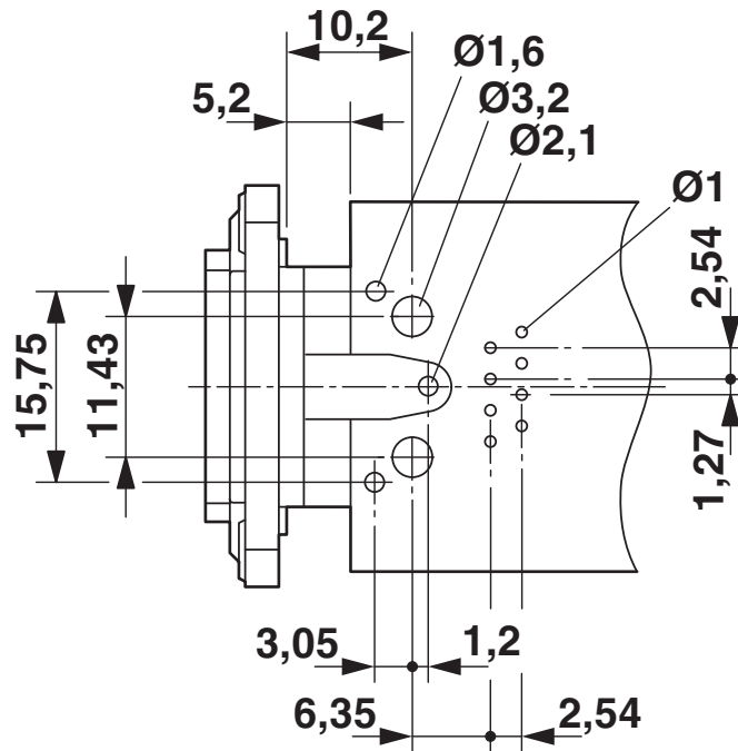
boorsjabloon/soldeerpadgeometrie
