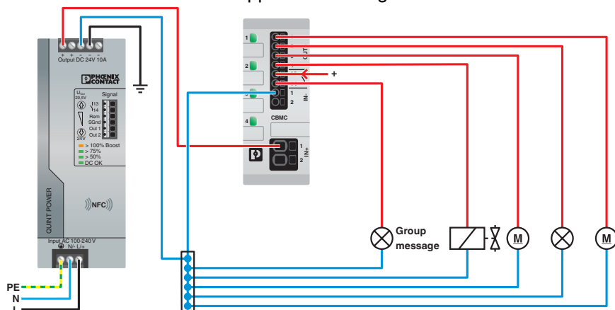
applicatietekening
