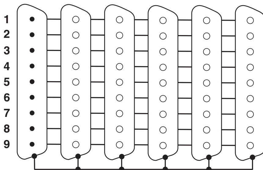
schakelschema
