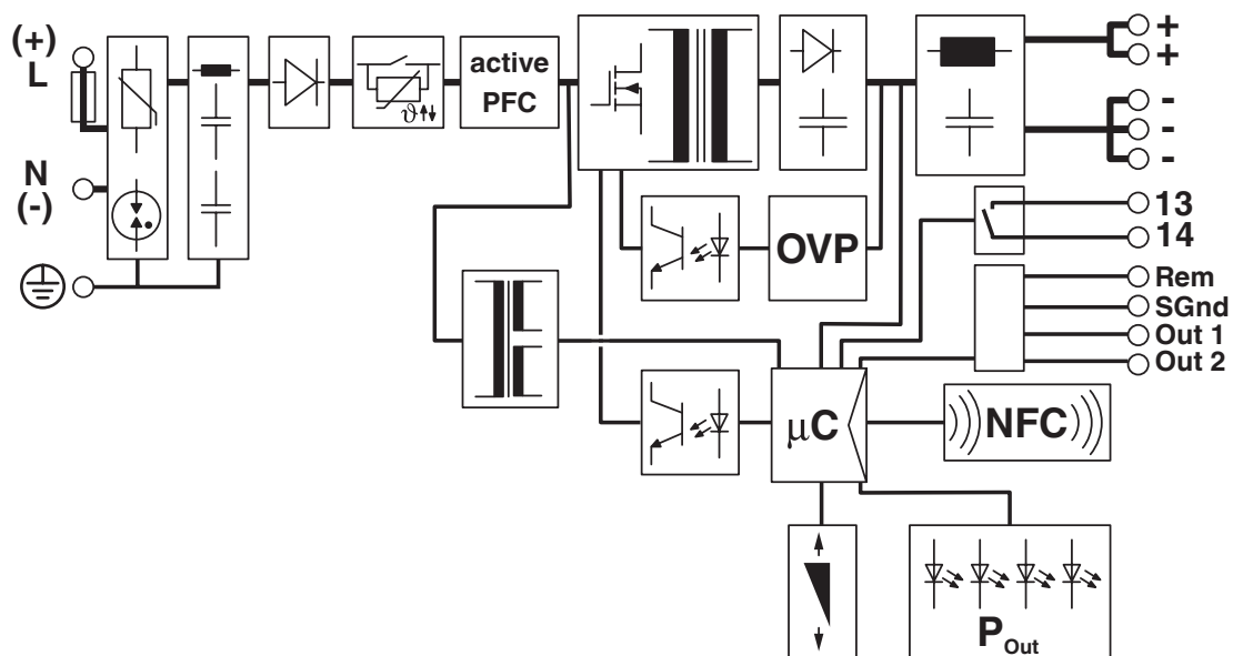
blokschema
