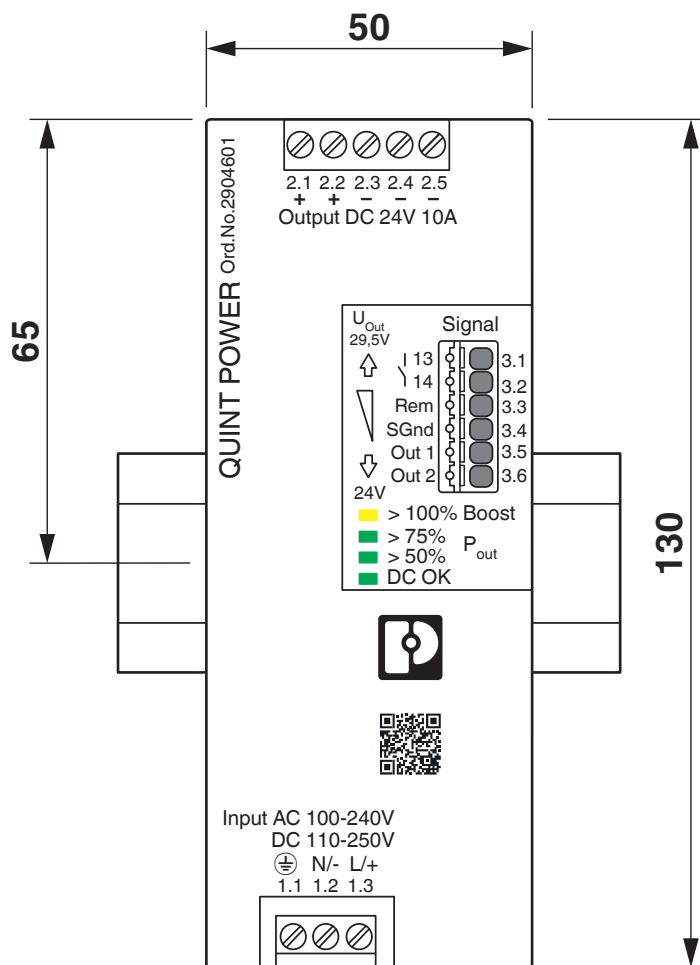
Maatschets
