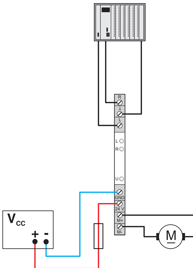
applicatietekening
