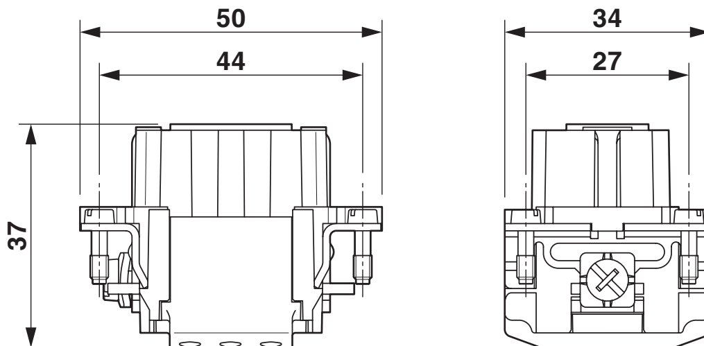
Maatschets
