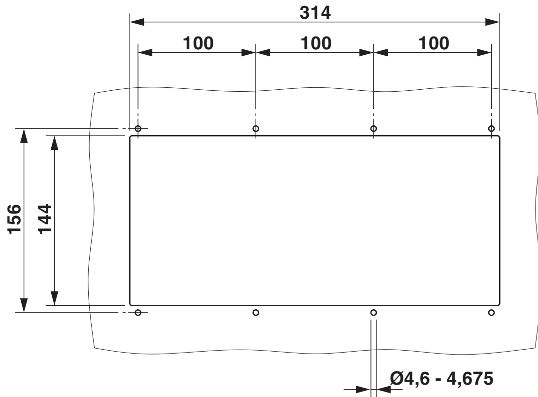
Tekening wanduitsparing
