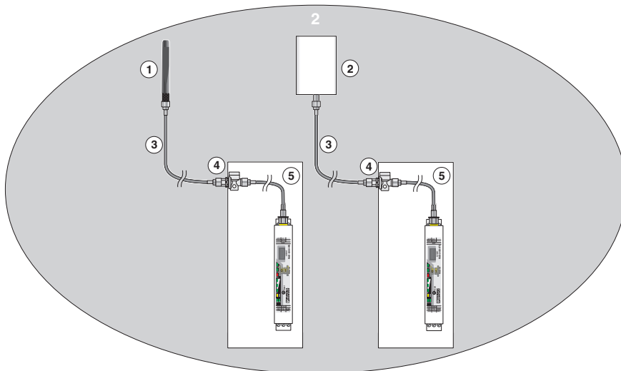
Installatie van apparaten en antennes in zone 2
