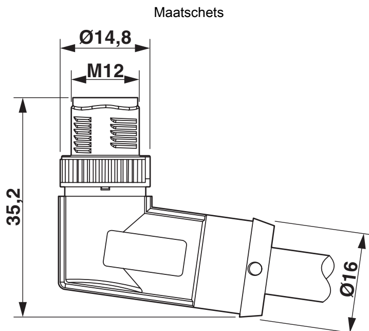
schematekening
