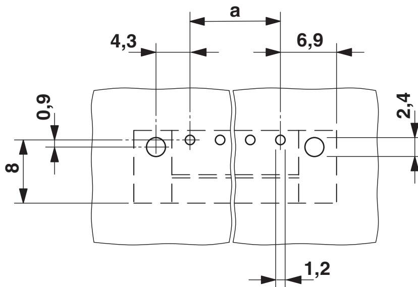
boorsjabloon/soldeerpadgeometrie
