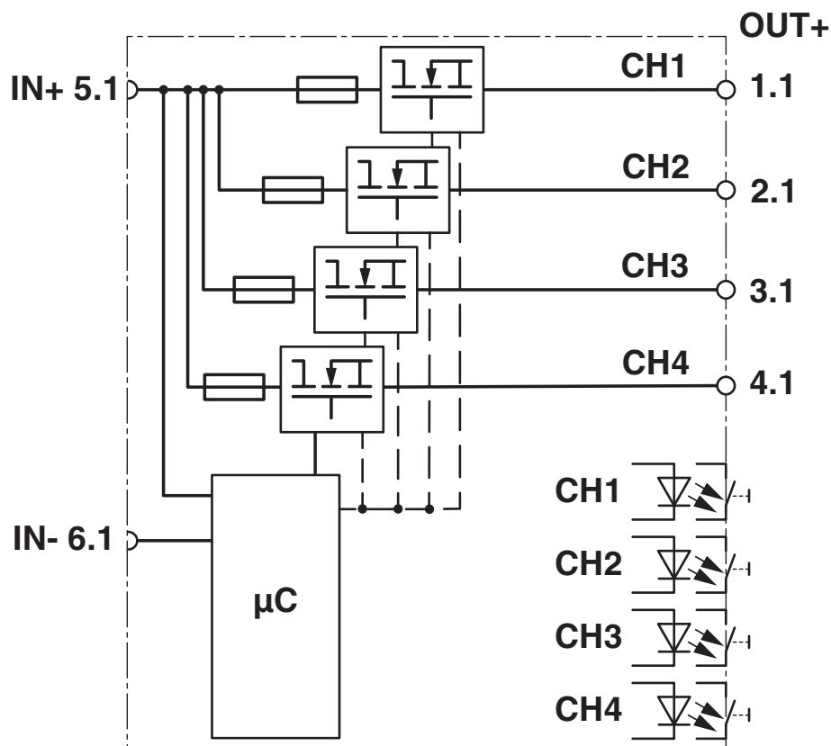
blokschema
