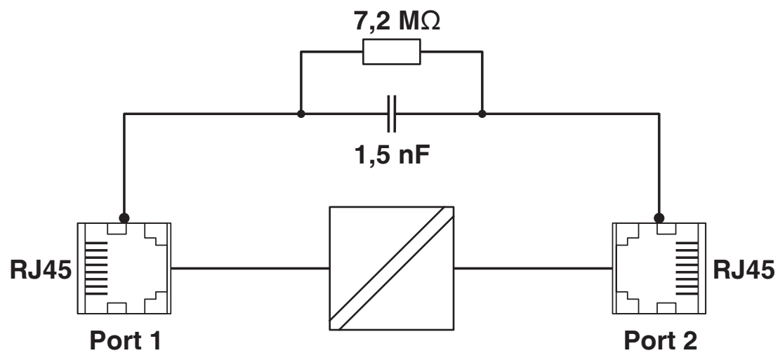
blokschema
