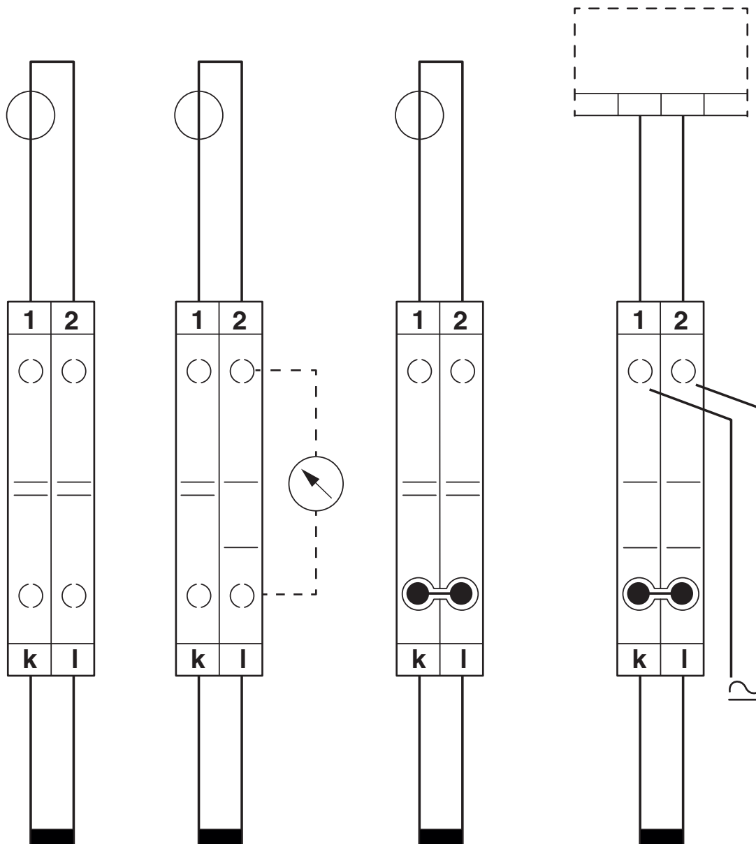
schematekening
