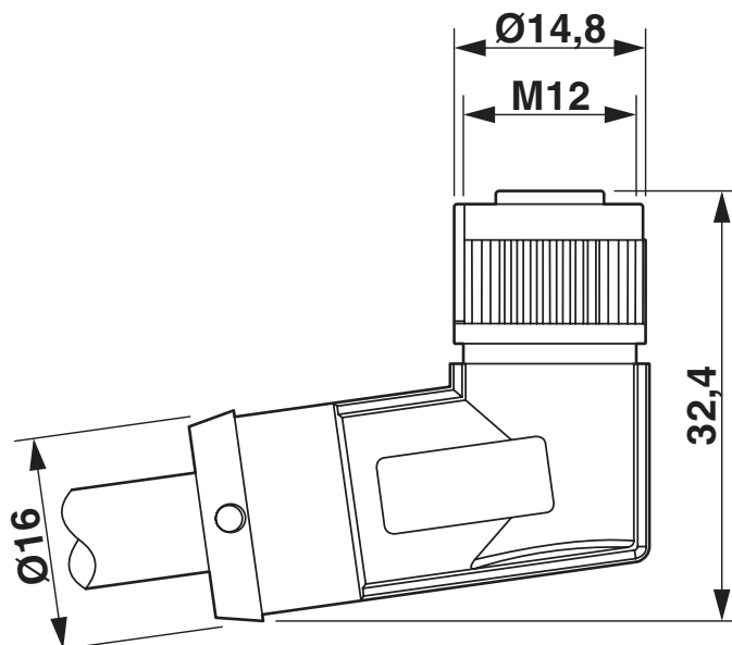
Maatschets
