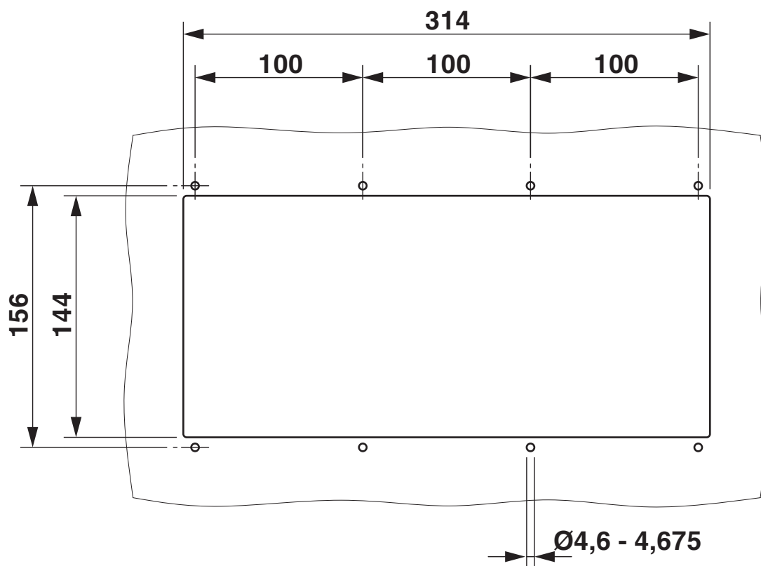
Tekening wanduitsparing
