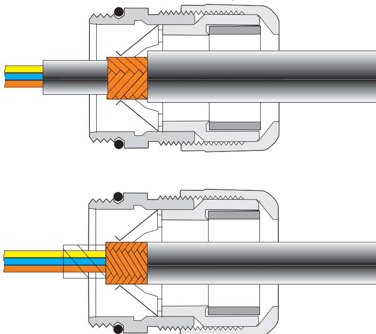
functietekening
