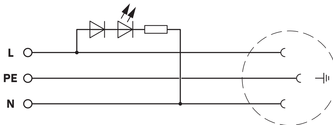
schakelschema
