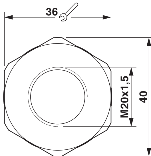
Maatschets
