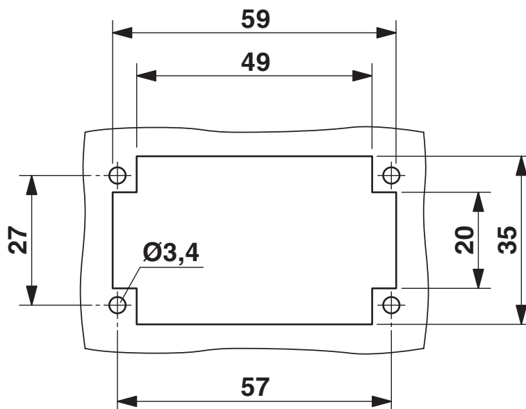
Maatschets
