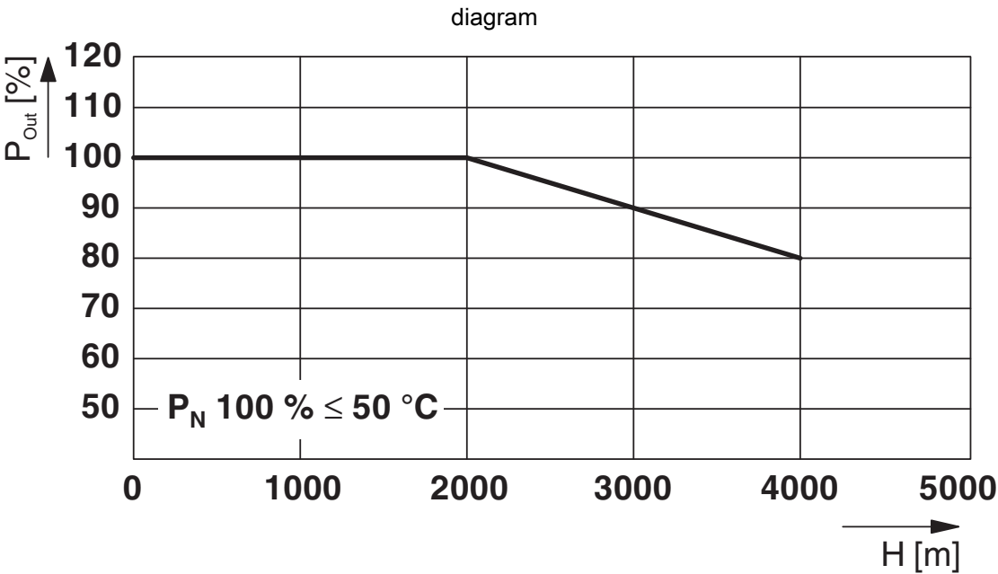
Uitgangsvermogen/opstelhoogte
