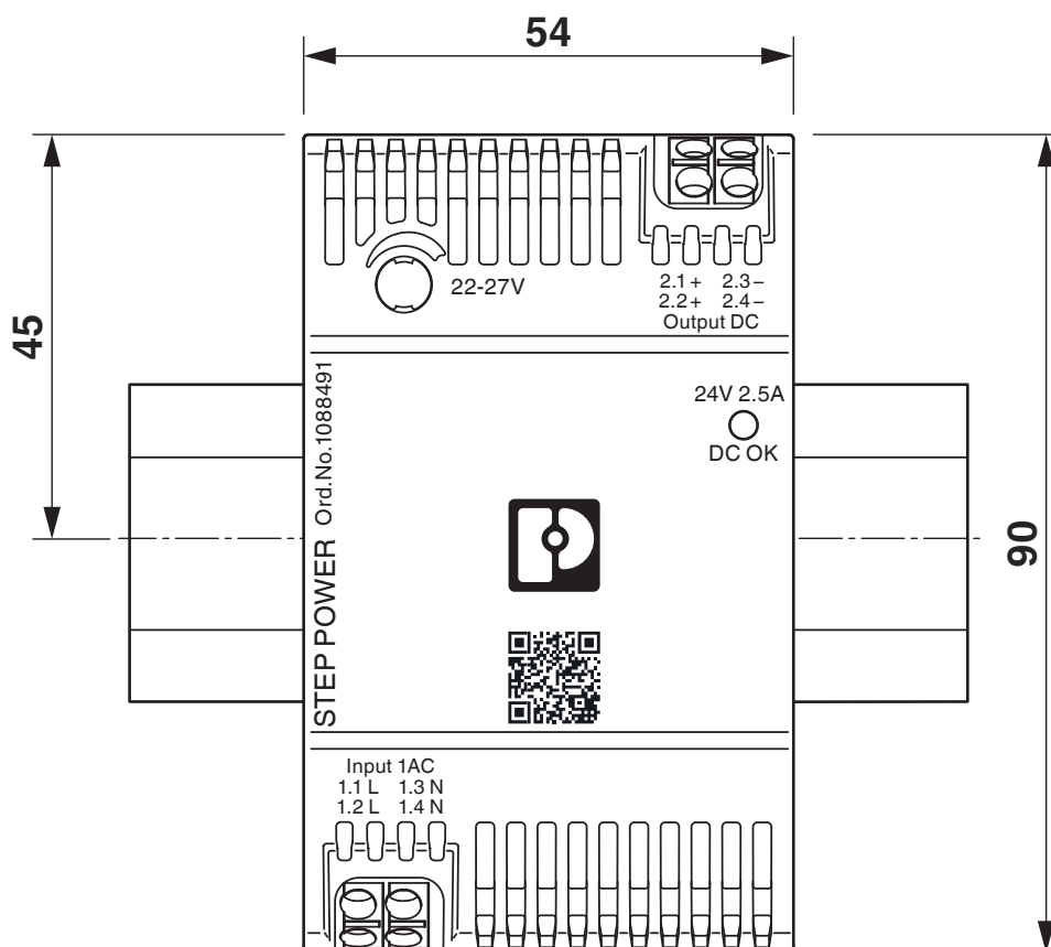
Maatschets
