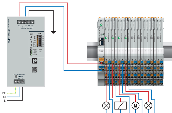
applicatietekening
