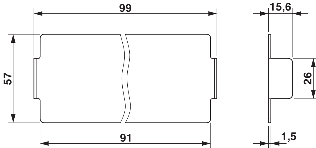
Maatschets
