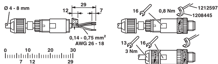
functietekening
