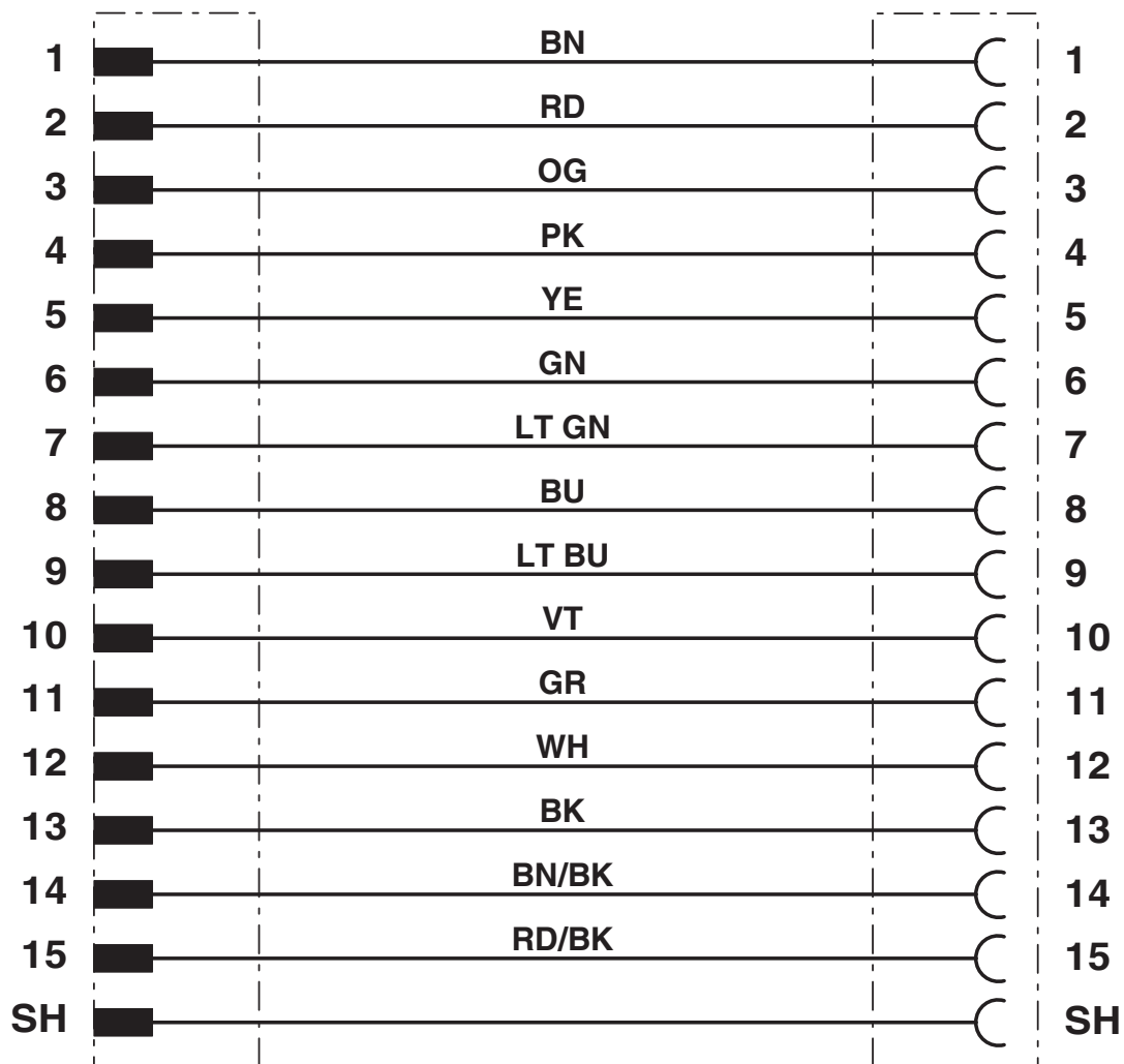
schakelschema
