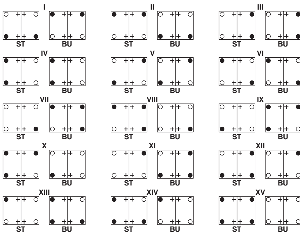
schematekening
