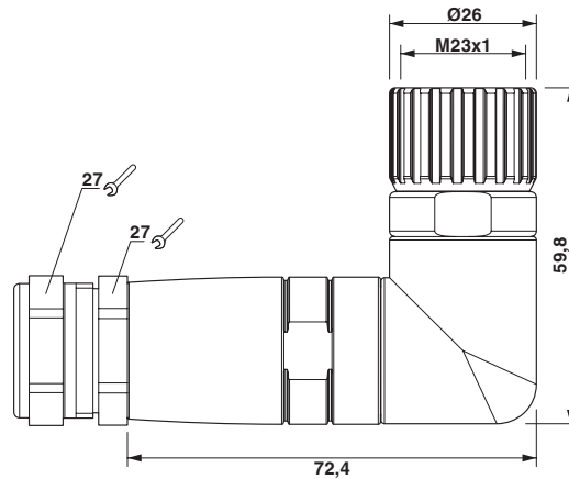
Maatschets
