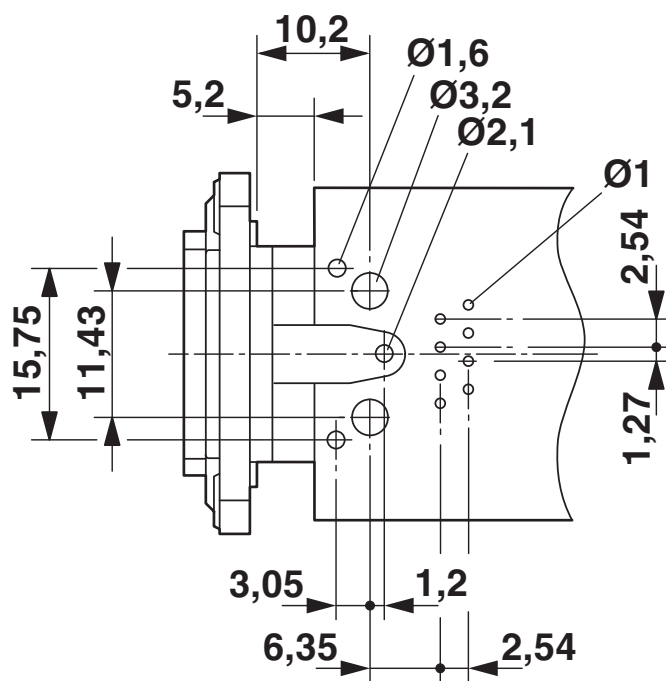
boorsjabloon/soldeerpadgeometrie
