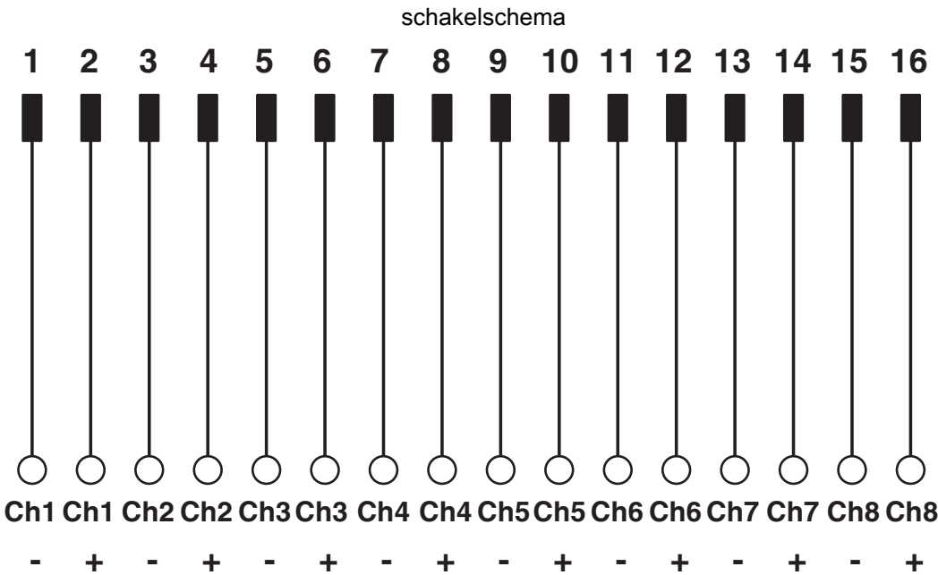
Aansluitschema FLKM 16/DV
