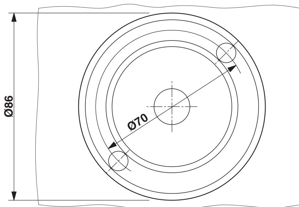
boorsjabloon/soldeerpadgeometrie
